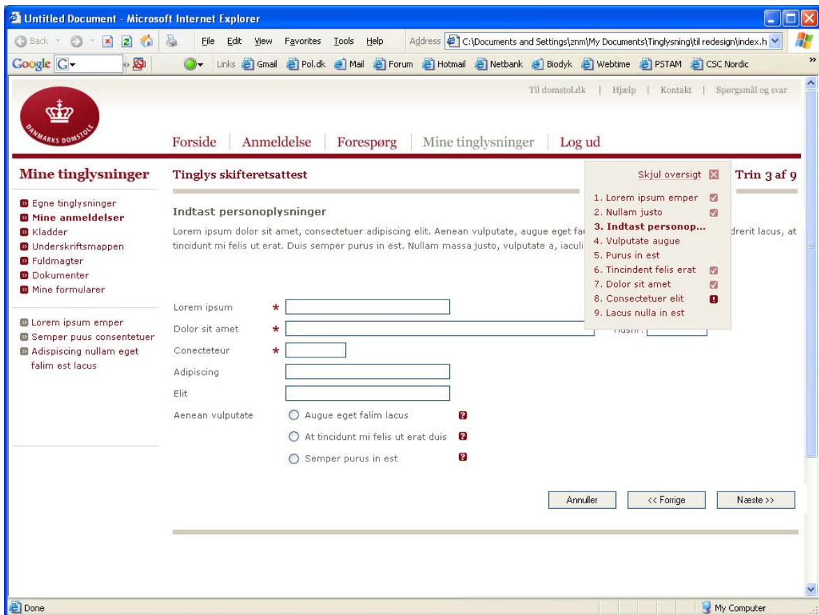
Figur 32 - Sideeksempel m. guide og formular
